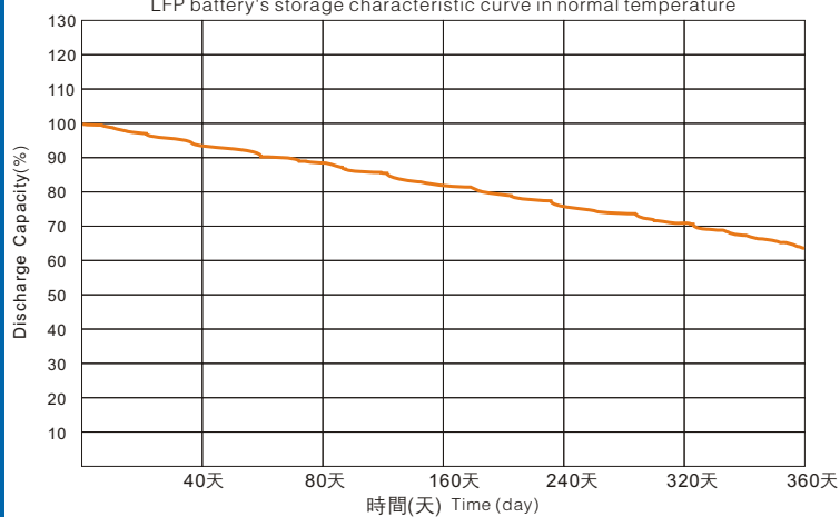
在常溫境溫下LFP類電池的存儲特性曲線
