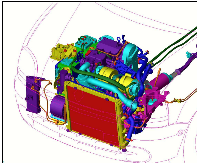
Vue du compartiment moteur
