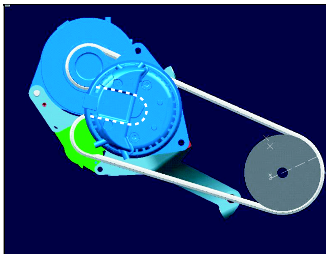
Vue de la courroie d'entraînement
