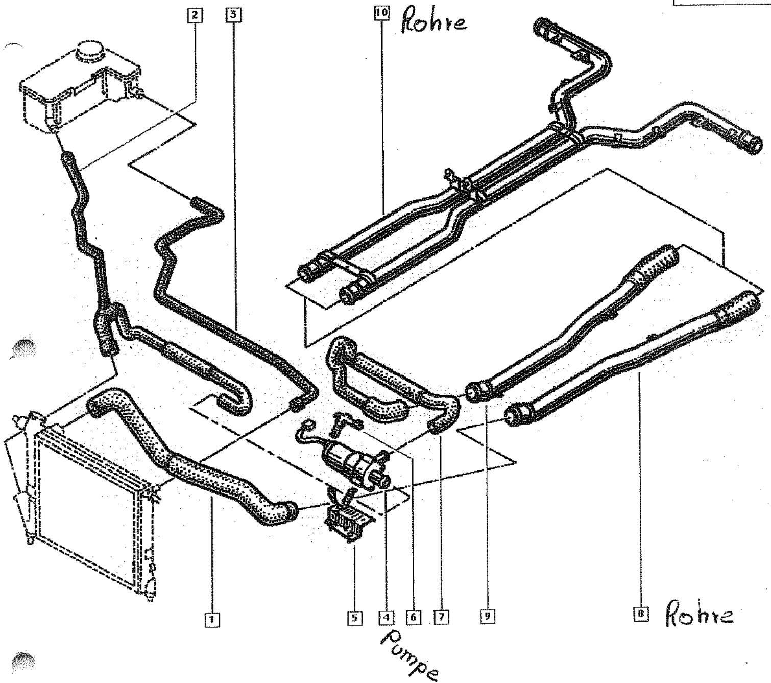
Kühlsystem der Fahrbatterien
